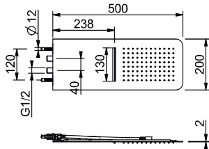
DIFUSOR 200 MM
