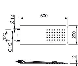
DIFUSOR 200 MM
