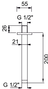
DIFUSOR DIÁMETRO 200 MM
